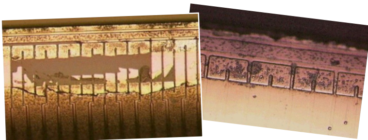
Beispiele eines durch ein minderwertiges Farbband zerstörten Druckkopfes
